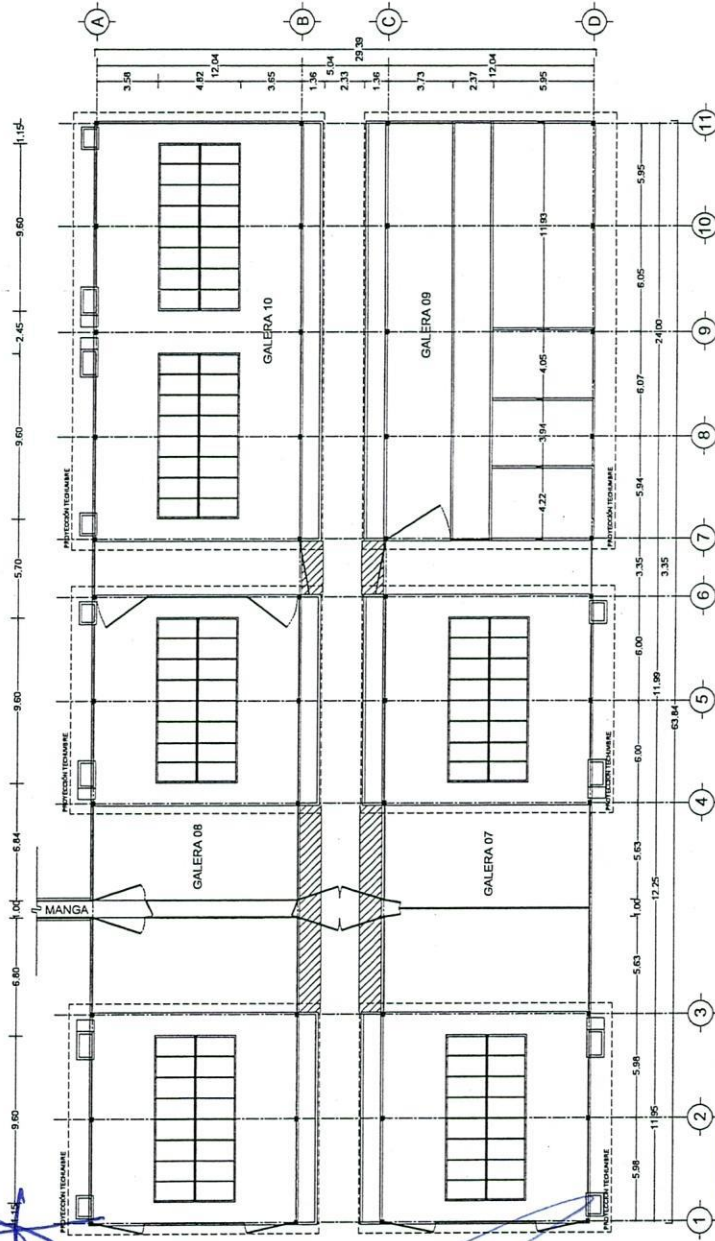
PLANTA ARQUITECTÓNICA GALERAS DE GANADO VACUNO
