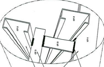
DT-02 DETALLE DE UNION DEL PERFIL CF-1, CF-2 Y CF-3 EN EL AREA DEL CABELETE
